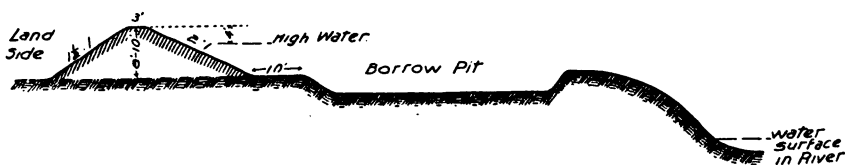
FIG. 91.—Specified section of Brevoort levee.
