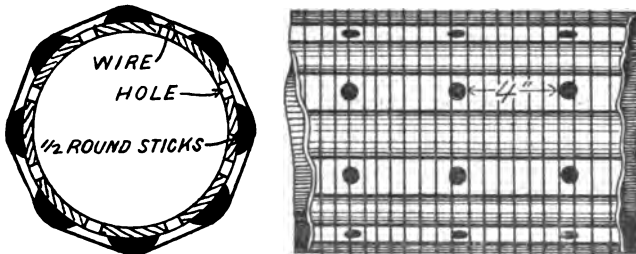
FIG. 48.—Strainer.
